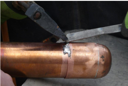
Verlöten der Kupferhülse
